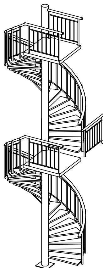
mehrstöckig, linksgewendelt
